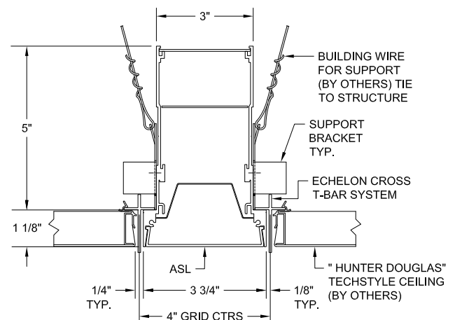
Echelon Cross T Bar: Specify EXSW code in catalog #
