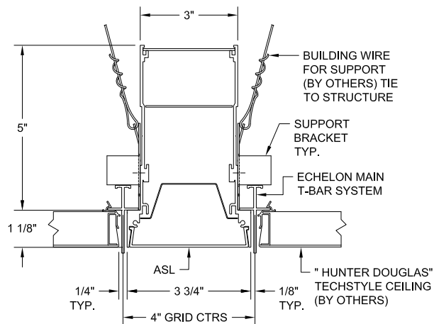
Echelon Main T Bar: Specify EMSW code in catalog #
