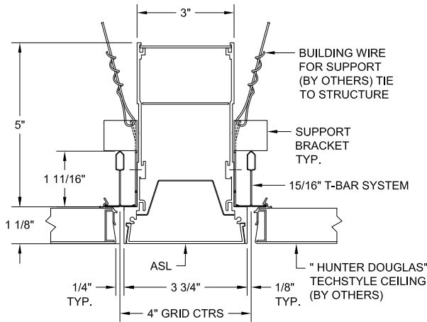
15/16" T Bar - 1 11/16": Specify T1SW code in catalog #
