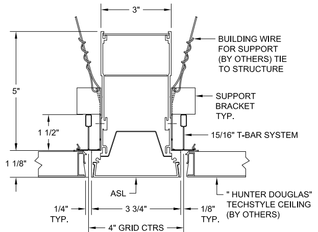
15/16" T Bar - 1 1/2": Specify T1SW code in catalog #
